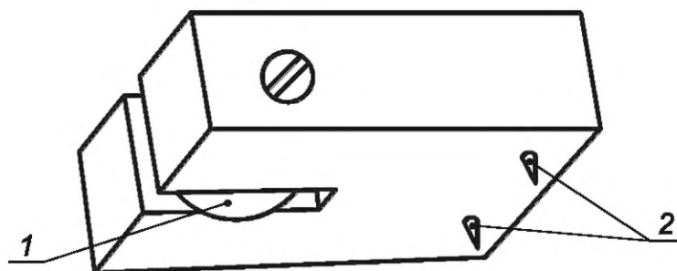
1 — индентор; 2 — опоры
